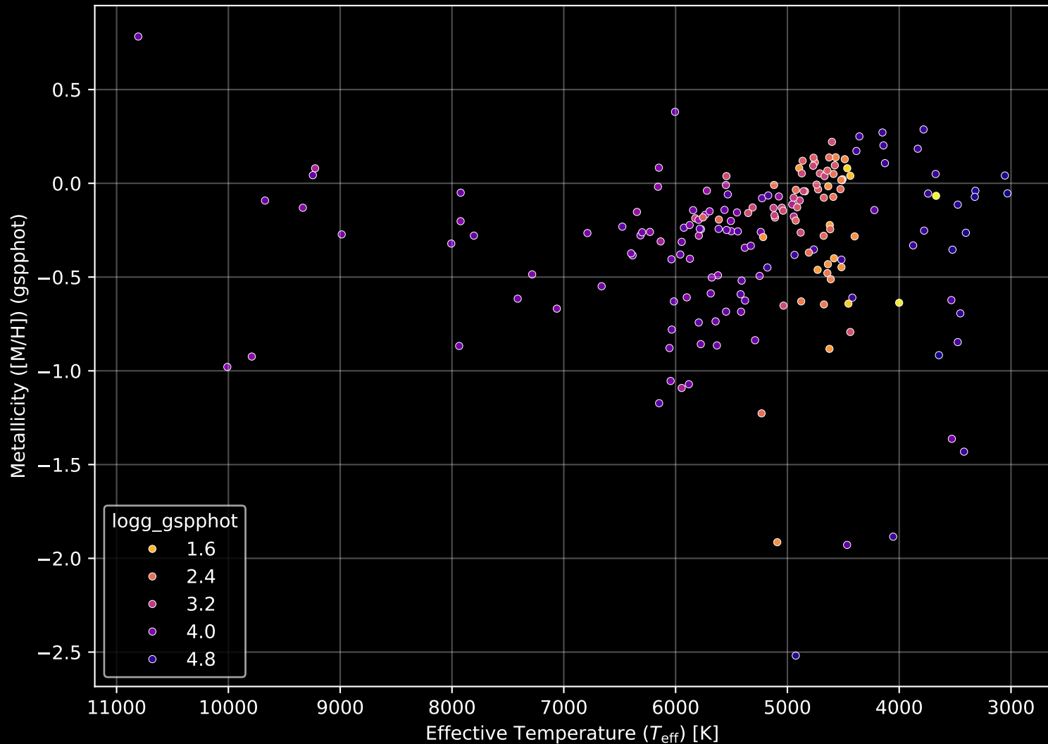
APOGEE DR17 Field: [K2_C7_012-13_btx] Stellar Population Parameters (n= 183)
